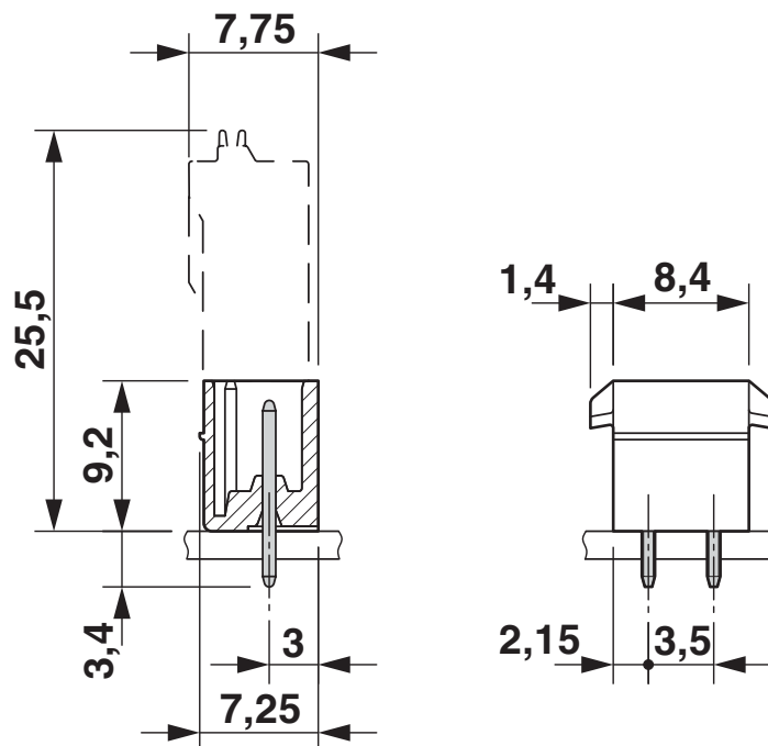
尺寸图
