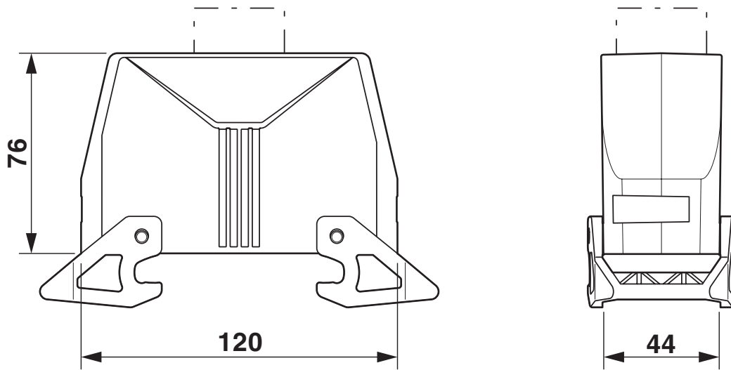
尺寸图
