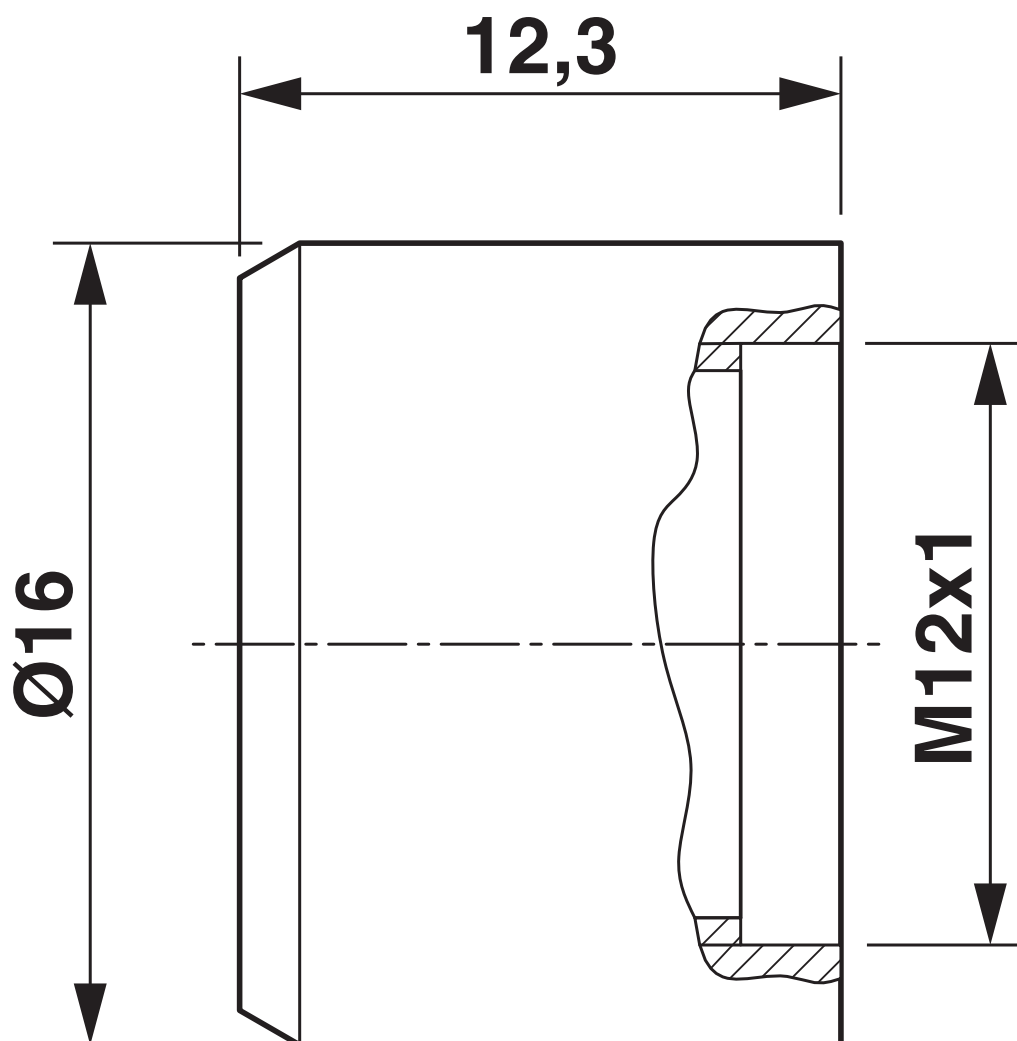
尺寸图
