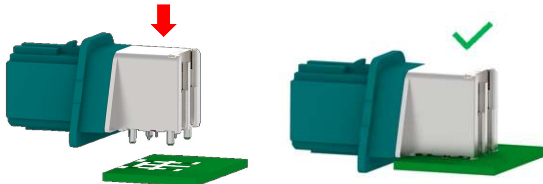
Fig.3 Pin Header 90° TE-NO. 2404815
