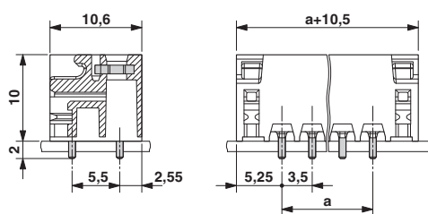
外形寸法
