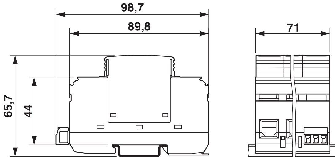
尺寸图
