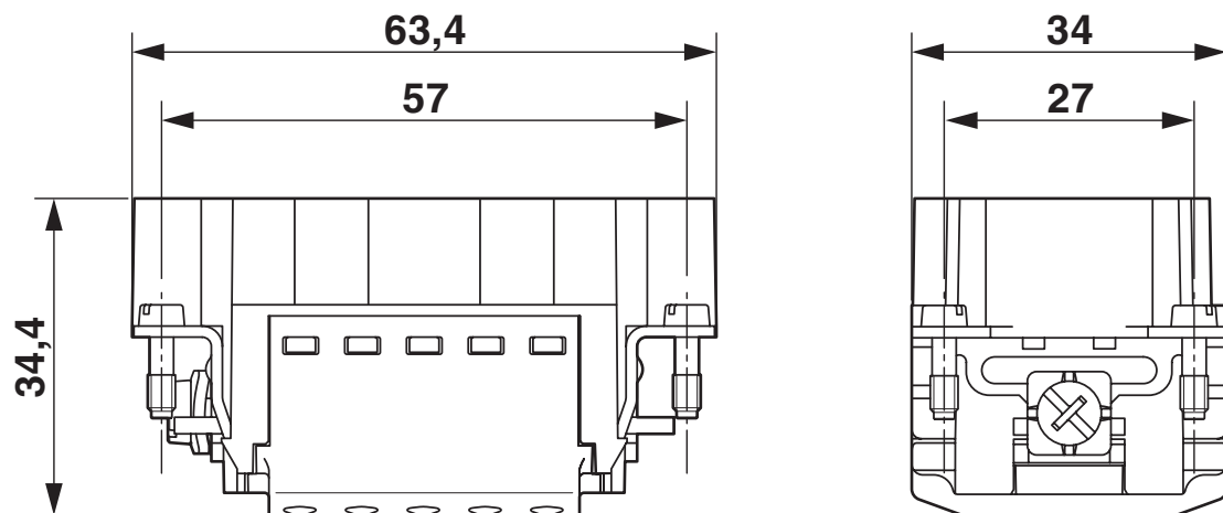
尺寸图
