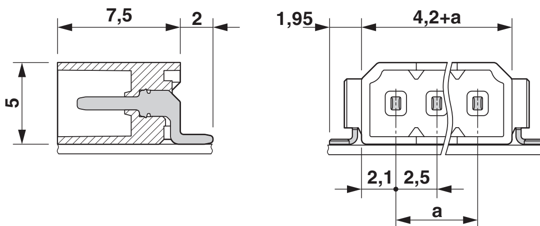
尺寸图
