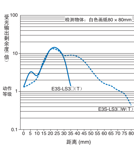
受光输出—距离特性
