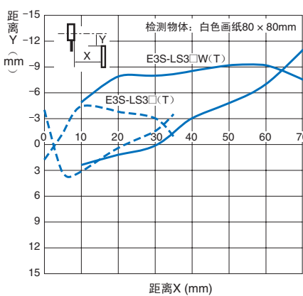
光点直径—距离特性 (E3S-LS3(T)、E3S-LS3W(T)共通)
