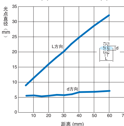
光点直径—距离特性 (E3S-LS3(T)、E3S-LS3W(T)共通)
