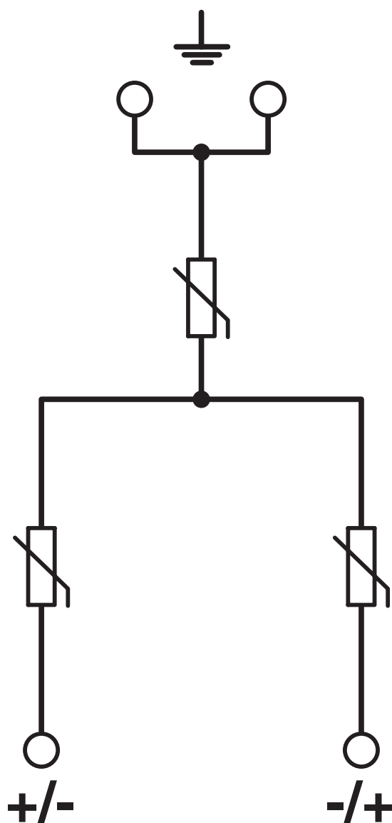
电路图
