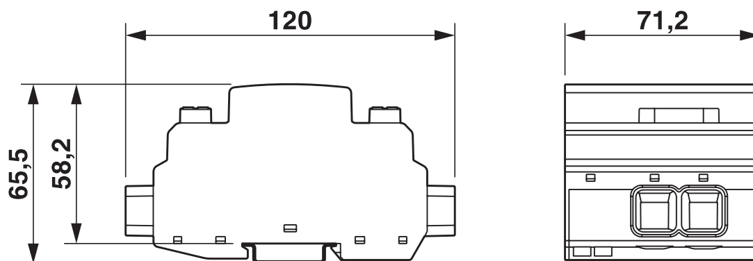
尺寸图
