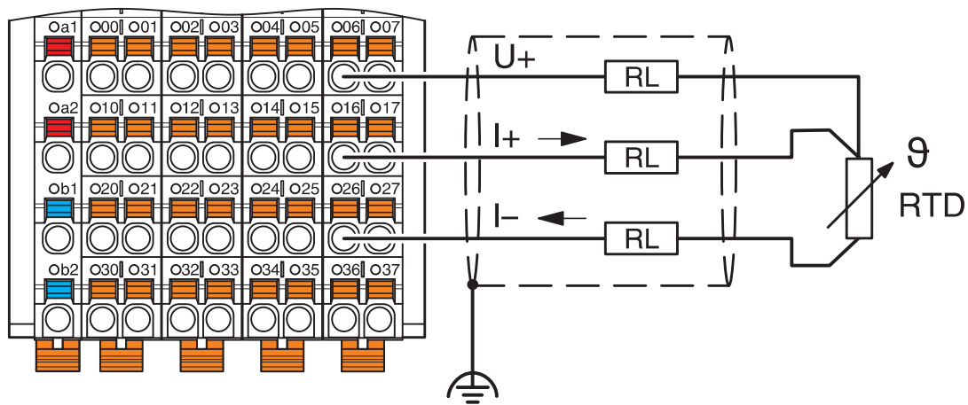
接线图
