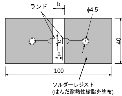
図1 (単位:mm)
