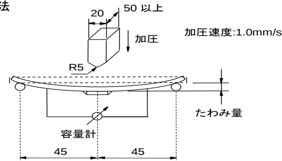
図2 (単位:mm)
