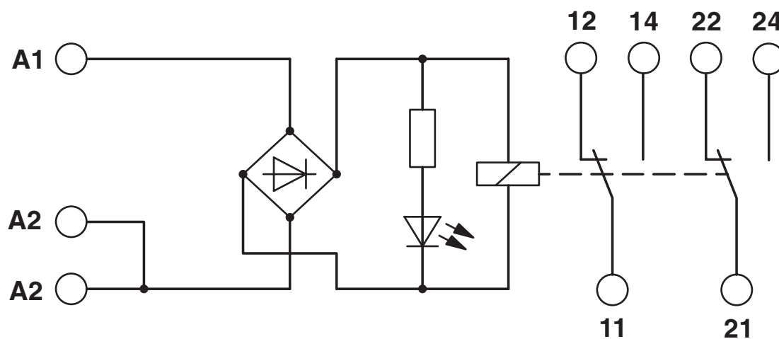
电路图
