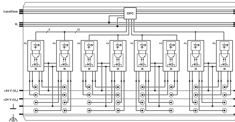
结构框图
