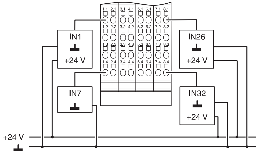
接线图
