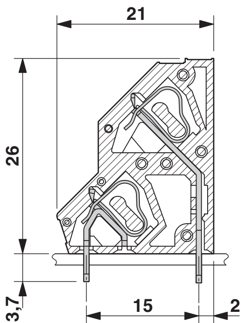
尺寸图
