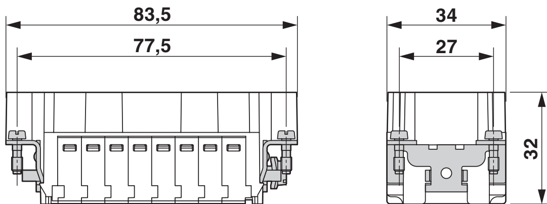
尺寸图
