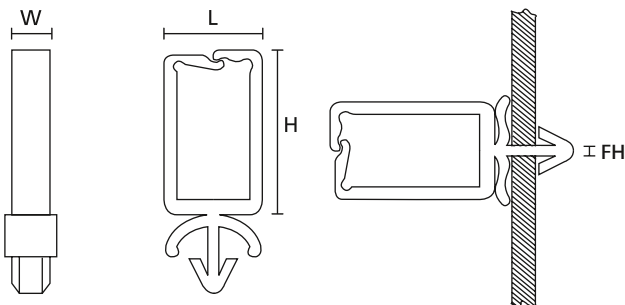
Kabelhalter WPC (Seitenansicht, Frontansicht und in der Anwendung)
