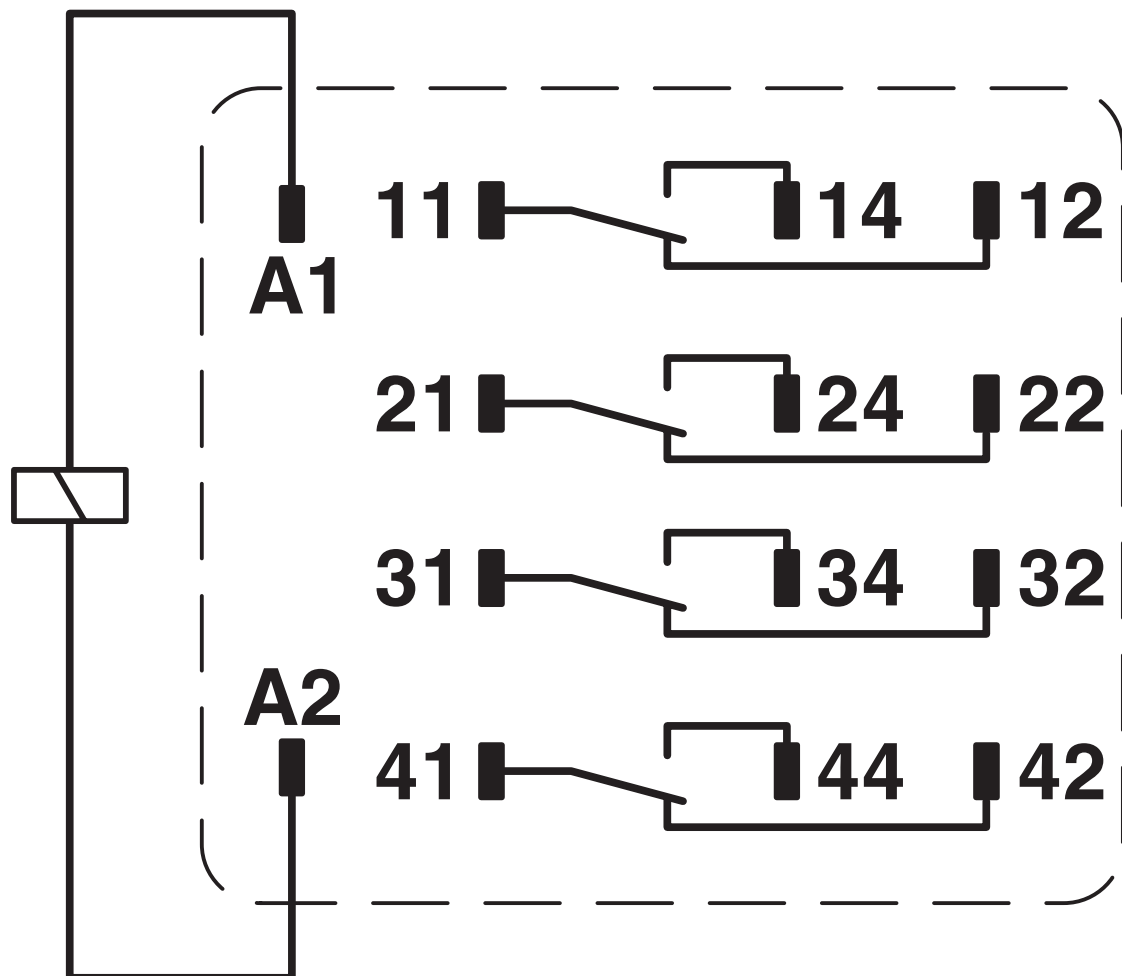
电路图
