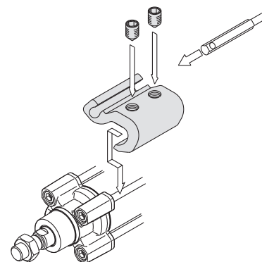
• Esempio di montaggio di D-A9□(V), M9□(V), M9□W(V), M9□A(V)
