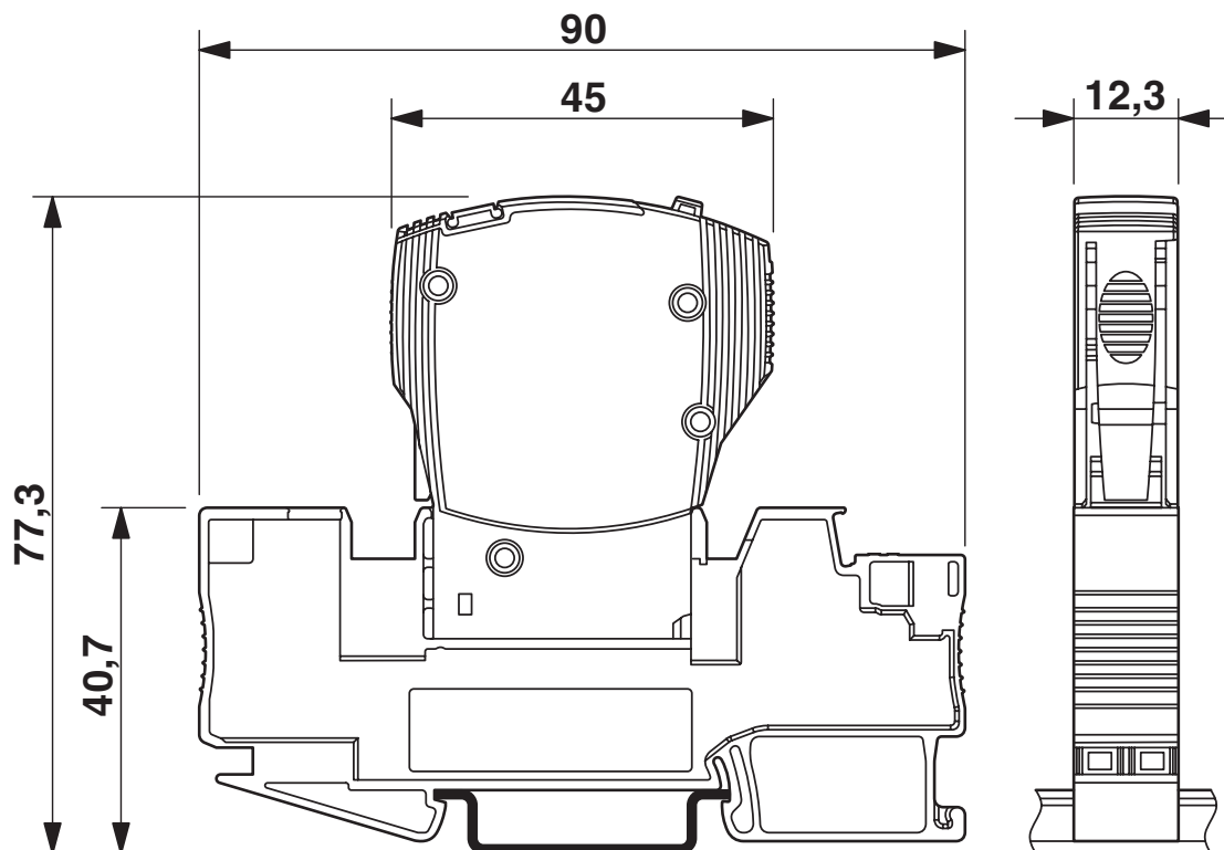
尺寸图
