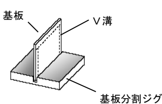
〔ジグ概要〕
