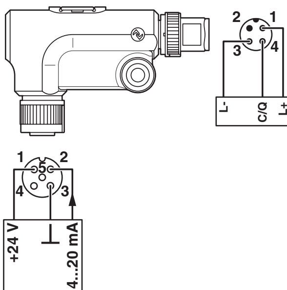
Anschlusszeichnung
