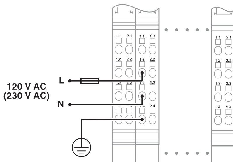
接线图
