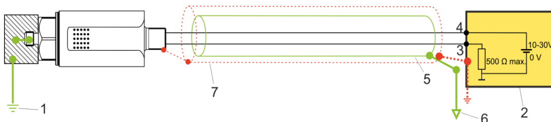
Fig. 10: Standardjordningskoncept
