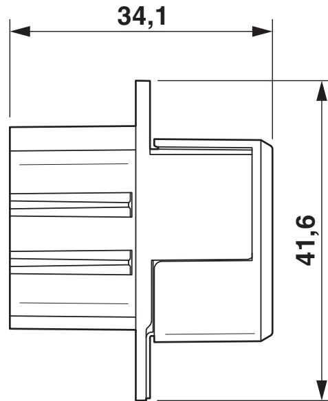
尺寸图
