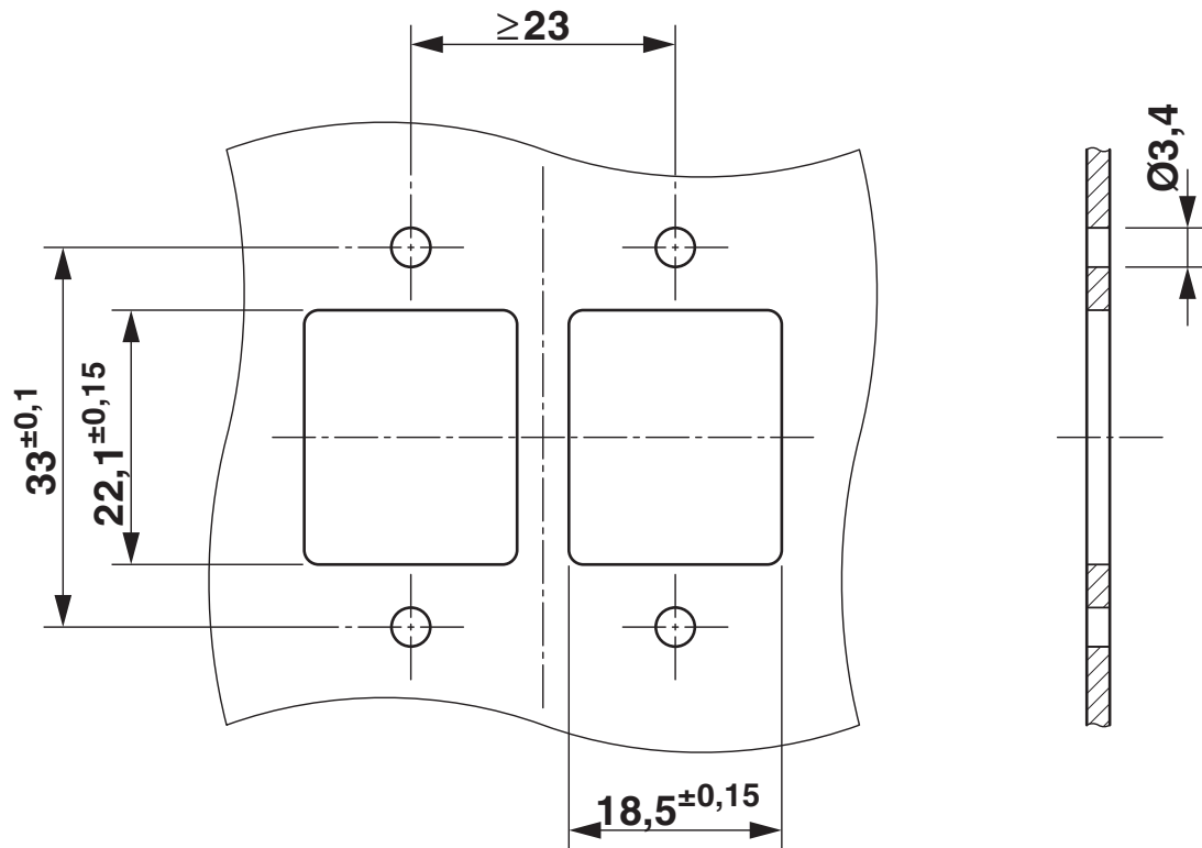
Bohrplan/Lötpadgeometrie
