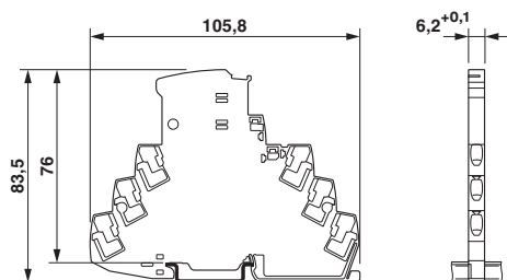
Dessin coté
