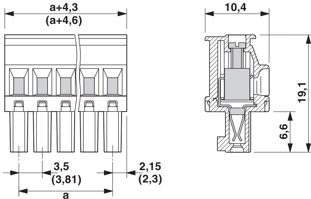
尺寸图
