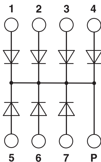
电路图
