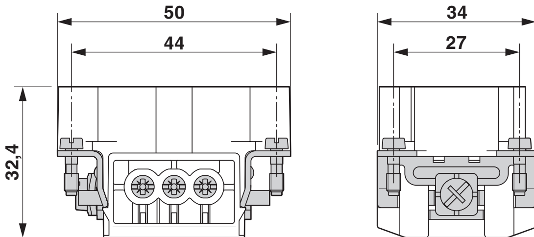
Maßzeichnung
