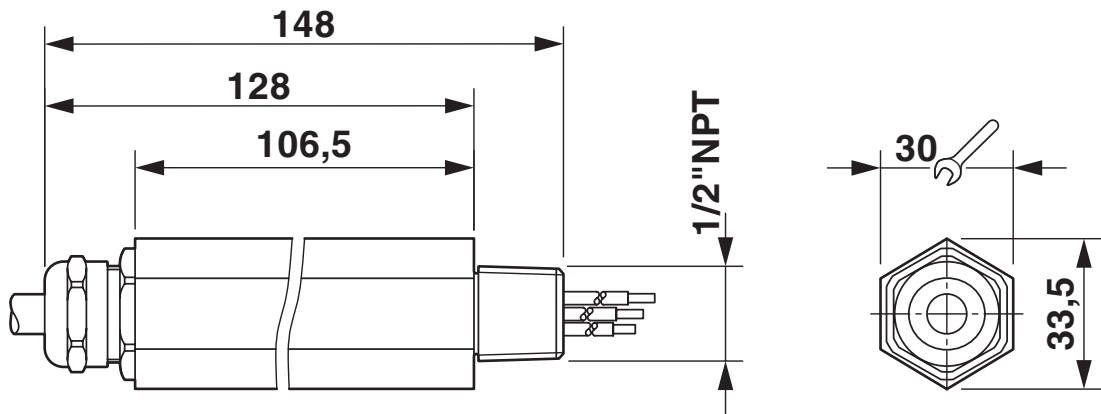
尺寸图
