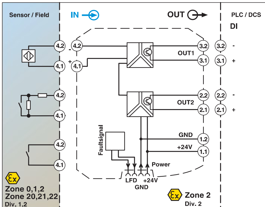
结构框图
