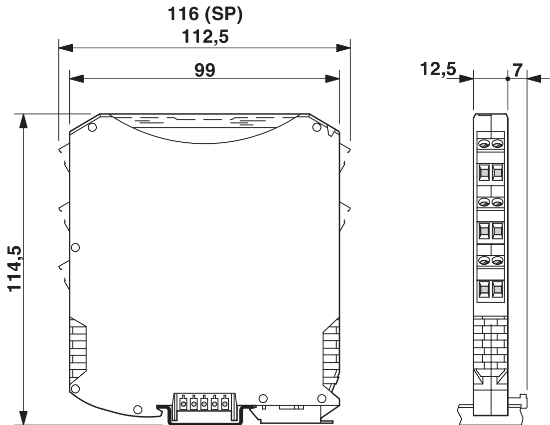
尺寸图
