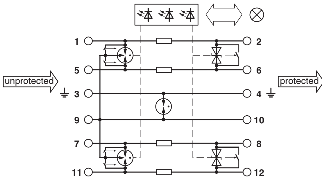
电路图
