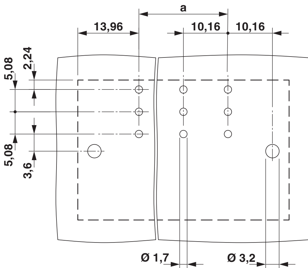
开孔图/焊盘环宽
