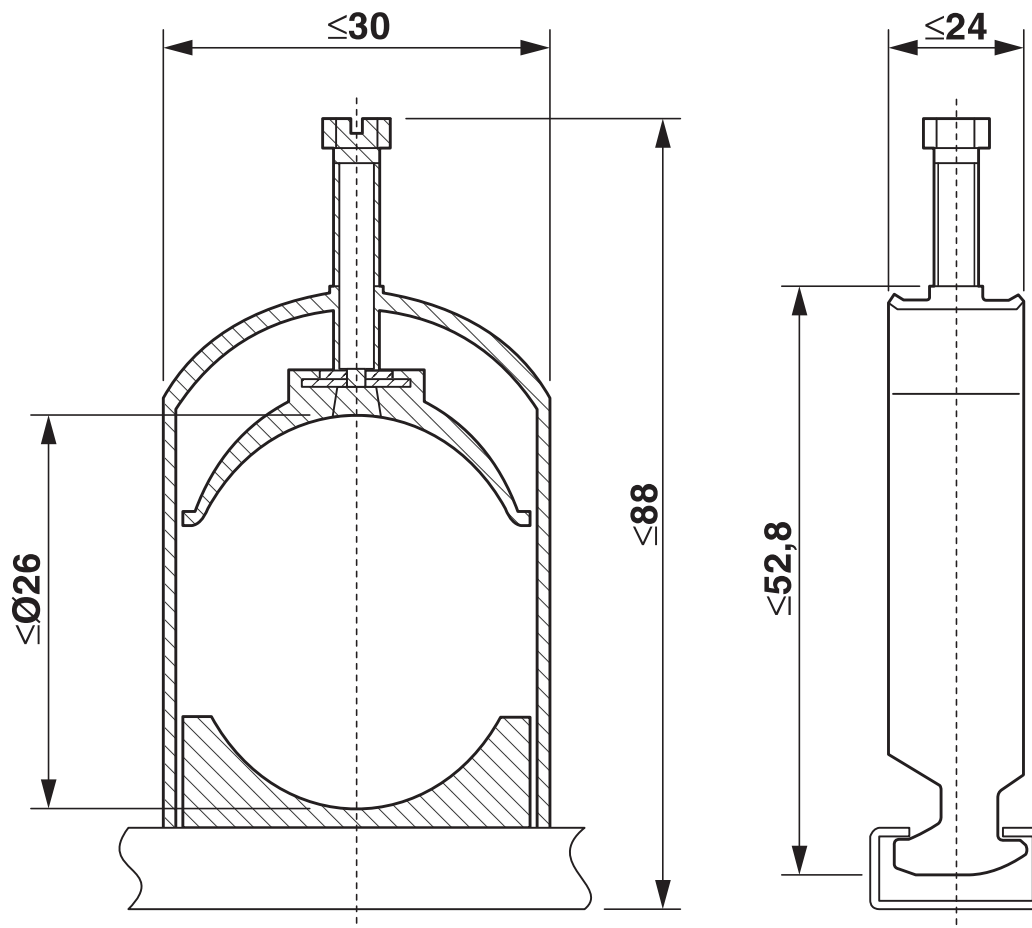
尺寸图
