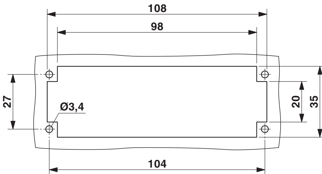
Montageausschnitt bei Verwendung ohne Gehäuse
