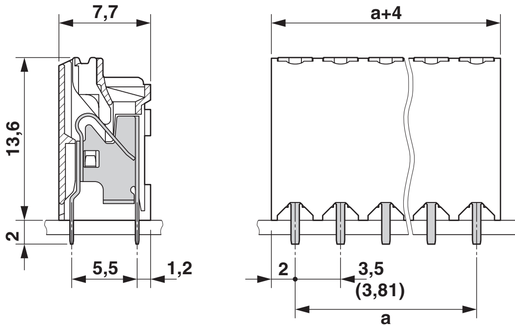
尺寸图
