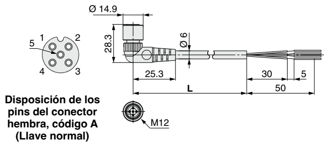
Modelo de conector en ángulo
