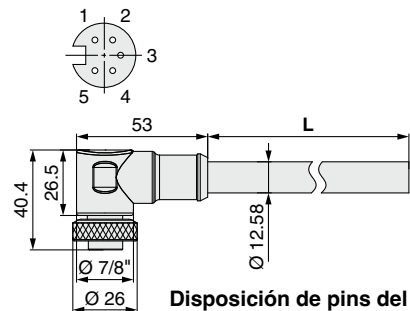
Disposición de pins del conector hembra
