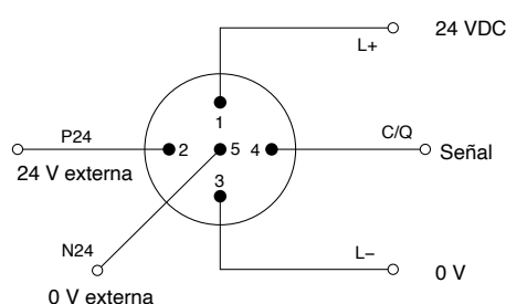
Clase de conexión B
