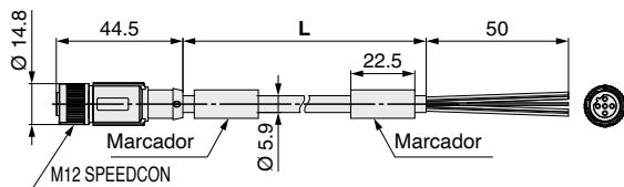
Modelo de conector recto
