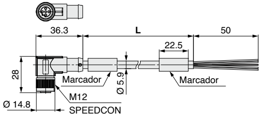
Modelo de conector en ángulo
