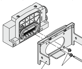
Placa de válvula Tornillo de sujeción de la válvula
