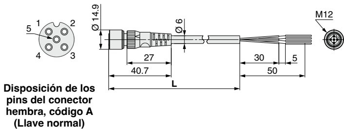
Modelo de conector recto
