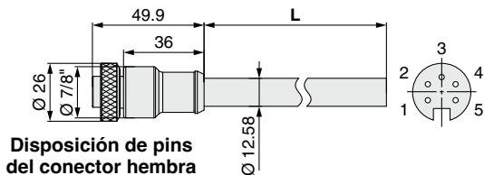
Modelo de conector recto
