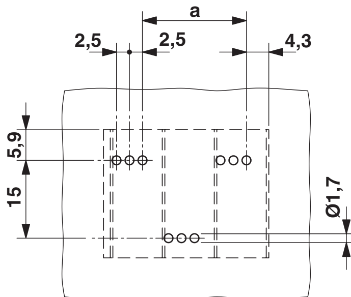
Bohrplan/Lötpadgeometrie
