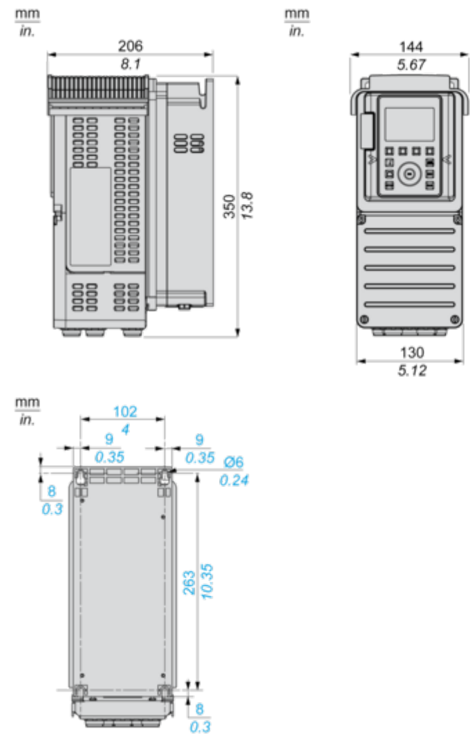
右侧、正面和背面视图
