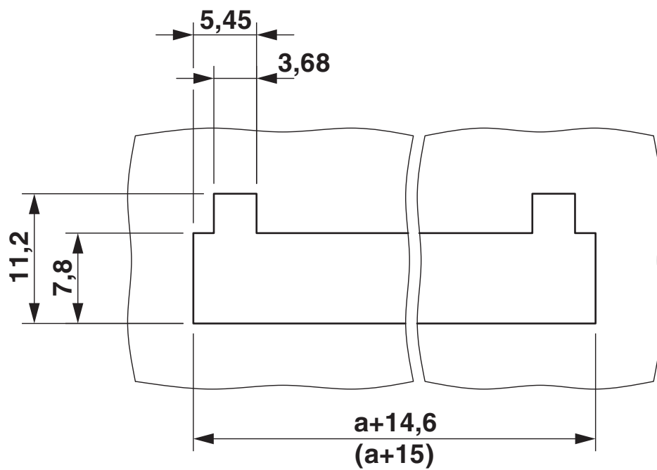
尺寸图
