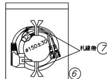
扎線示意图
