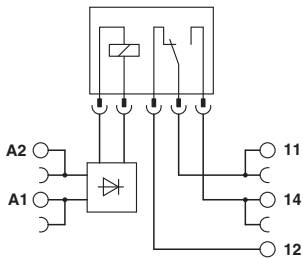
电路图
