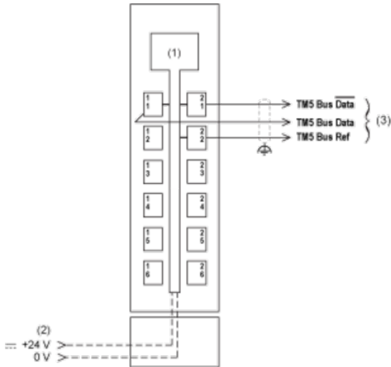
接线图
