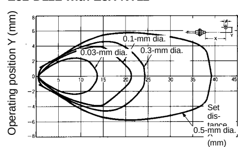
E32-D33 with E3X-NT11
