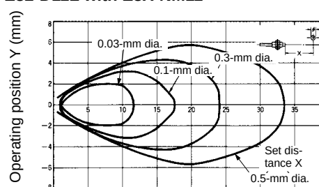
E32-D11L with E3X-NM11
