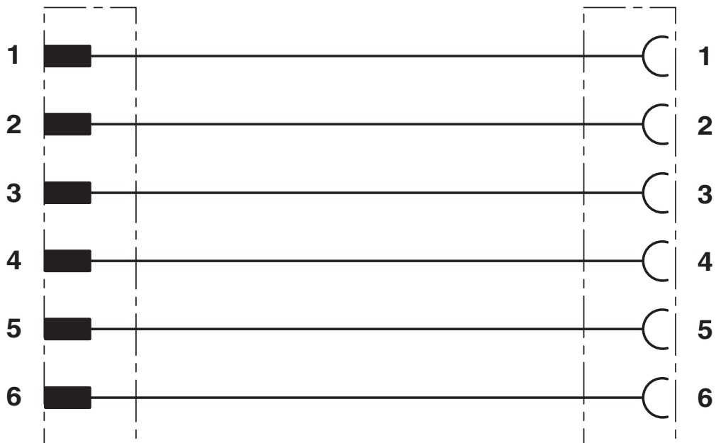
Schaltplan
