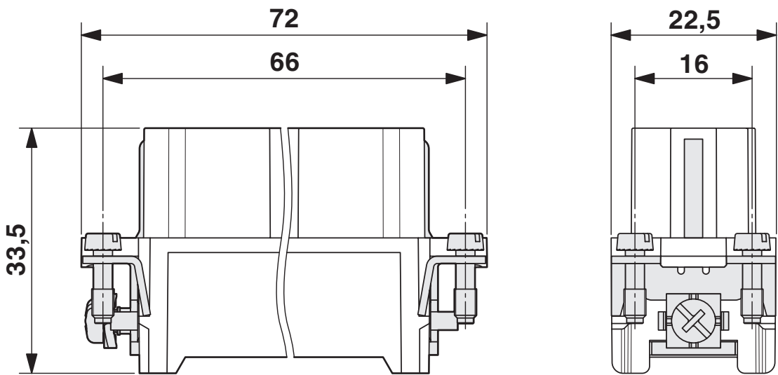
尺寸图
