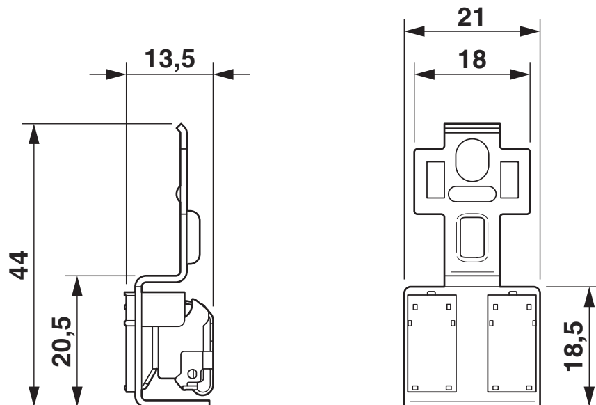
尺寸图
