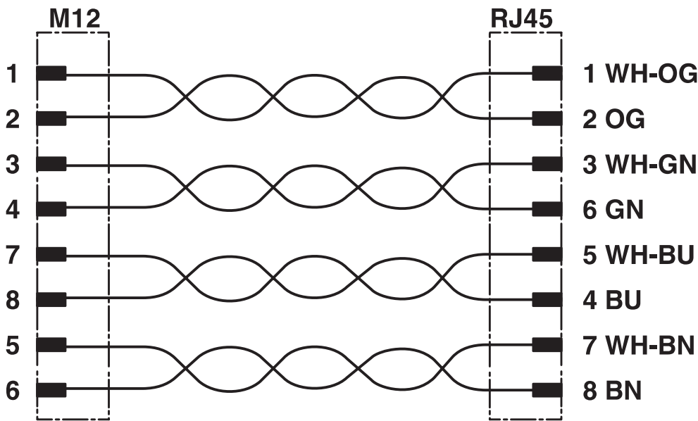
电路图
