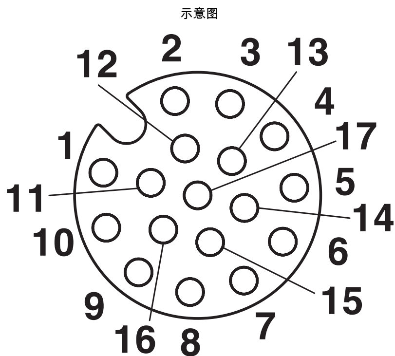
M12插座引脚分配，17芯，A编码，插座侧视图
